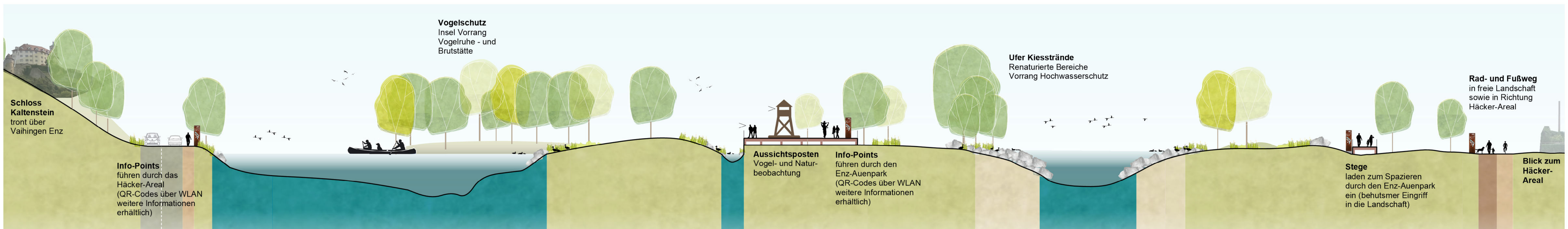
Schnitt Enz-Auenpark / M 1:250
