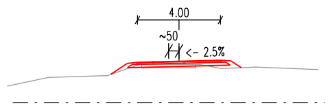
Querschnitt Radschnellweg
