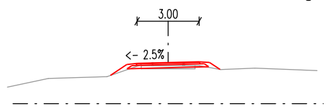
Querschnitt Geh- u. Radweg
